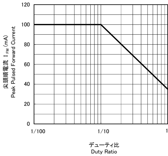
デューティ比 - 尖頭順電流 Peak Pulsed Forward Current vs. Duty Ratio ( T_C=25^\circ\text{C} )
